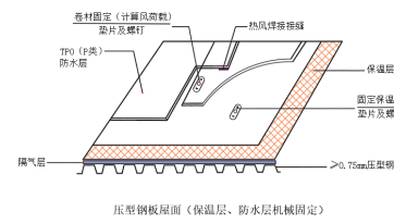
压型金属板屋面（保温层、防水层机械固定）
