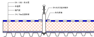
压型金属板屋面（光伏支架安装）
